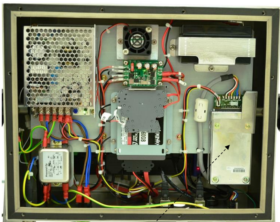
A/D Unit
