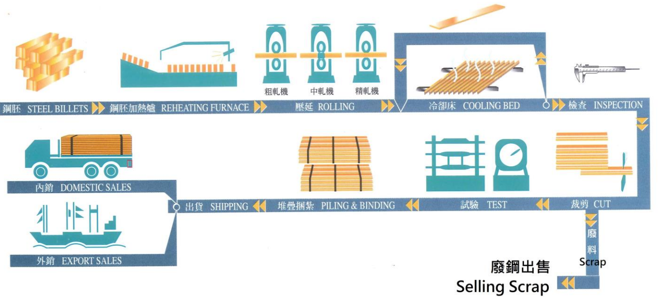
軋鋼設備生產流程圖 : Diagram of Rolling Steps
