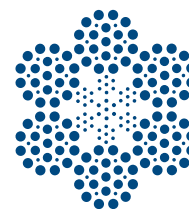
6x25 IWRC
