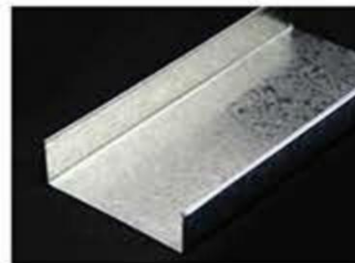
Metal Track (Hemmed) 52x28x28x3000 0.55BMT 0.490kg 65x28x28x3000 0.55BMT 0.545kg 77x28x28x3000 0.55BMT 0.599kg 93x28x28x3000 0.55BMT 0.665kg
