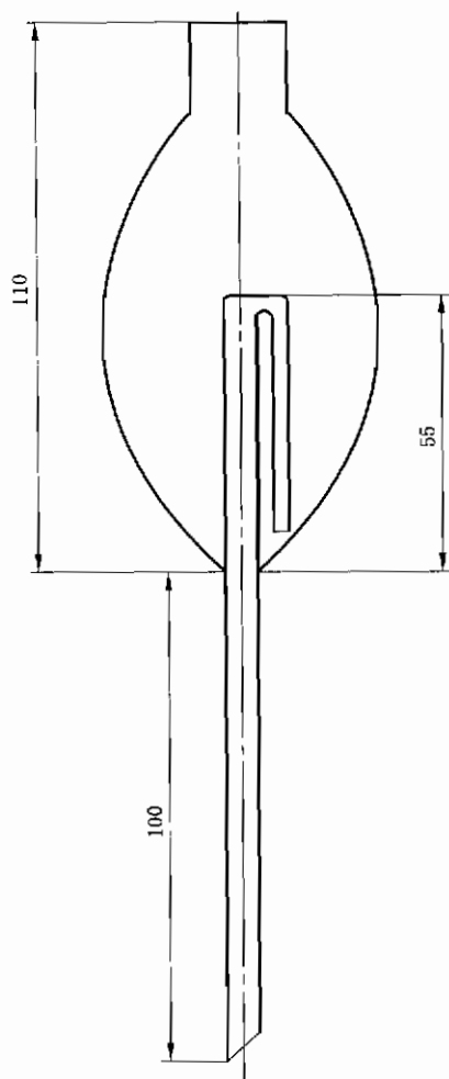
图 1 玻璃液封管
