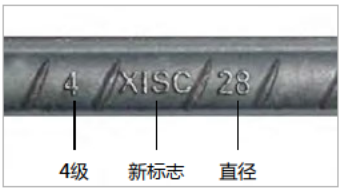
4级 新标志 直径
