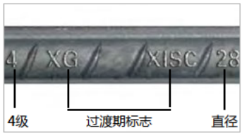
4级 过渡期标志 直径
